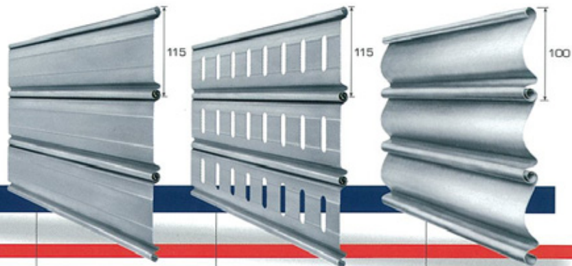
ELEMENTI PER SERRANDE DI GRANDI DIMENSIONI
